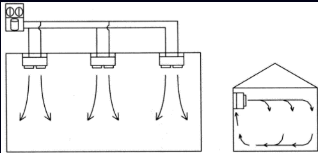
Placering af fordampere og rigtig dimensionering af køleanlægget gør, at der opnås en naturlig luftcirkulation i kølerummet.
